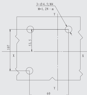
4P安装孔
