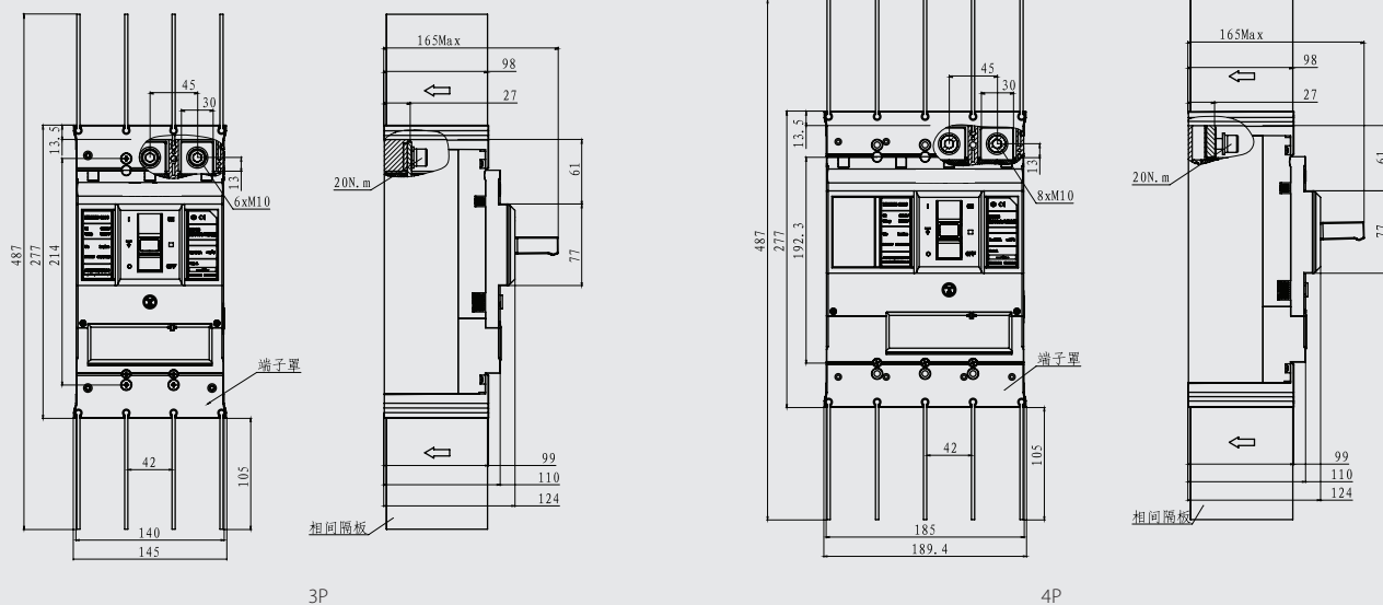
MDM5E-630 二维图
