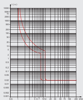
NDM5Z-1600 正常环境脱扣特性曲线 (800 A、1000 A)
