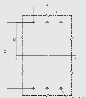
4P安装孔
