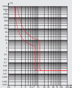
NDM5-1600脱扣曲线图 (800A、1000A)
