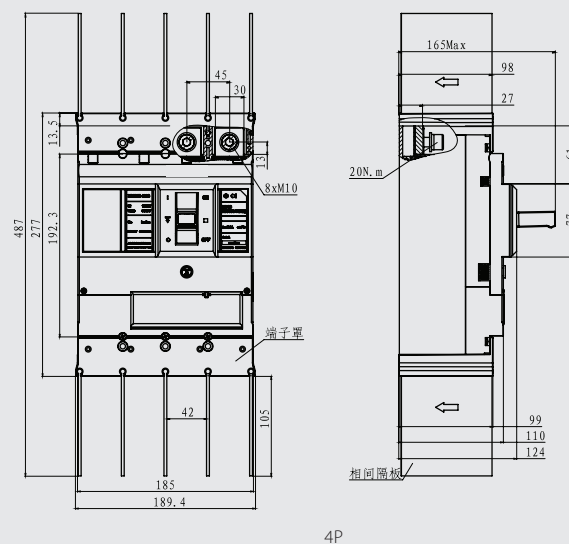
MDM5-630 二维图
