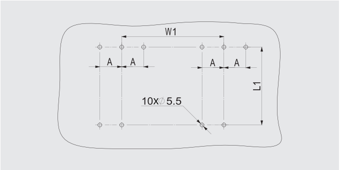
JS1机械联锁机构与断路器安装后的外形尺寸如下表所示，螺钉拧紧力矩值2N.m。（单位：mm）
