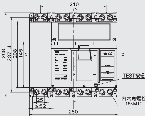
四极板前接线产品的外形尺寸
