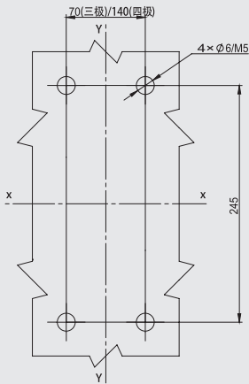
安装在底板上的安装开孔尺寸
