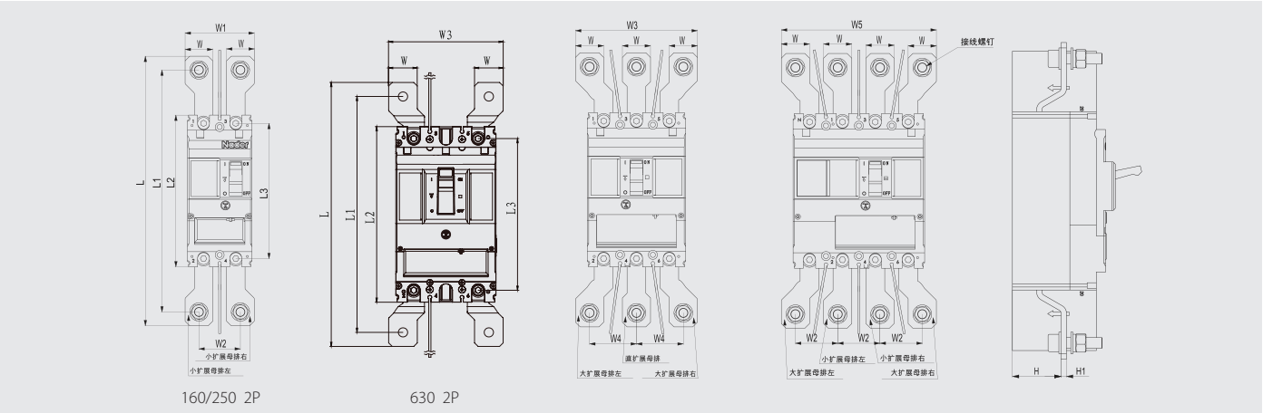
KM1板前接线扩展母排与断路器组合安装后的外形尺寸如下表所示：
