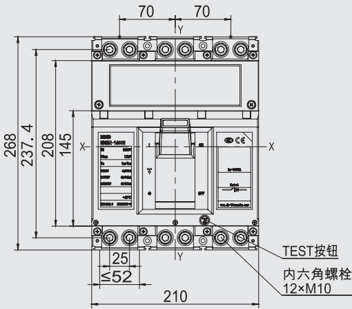
三极板前接线产品的外形尺寸
