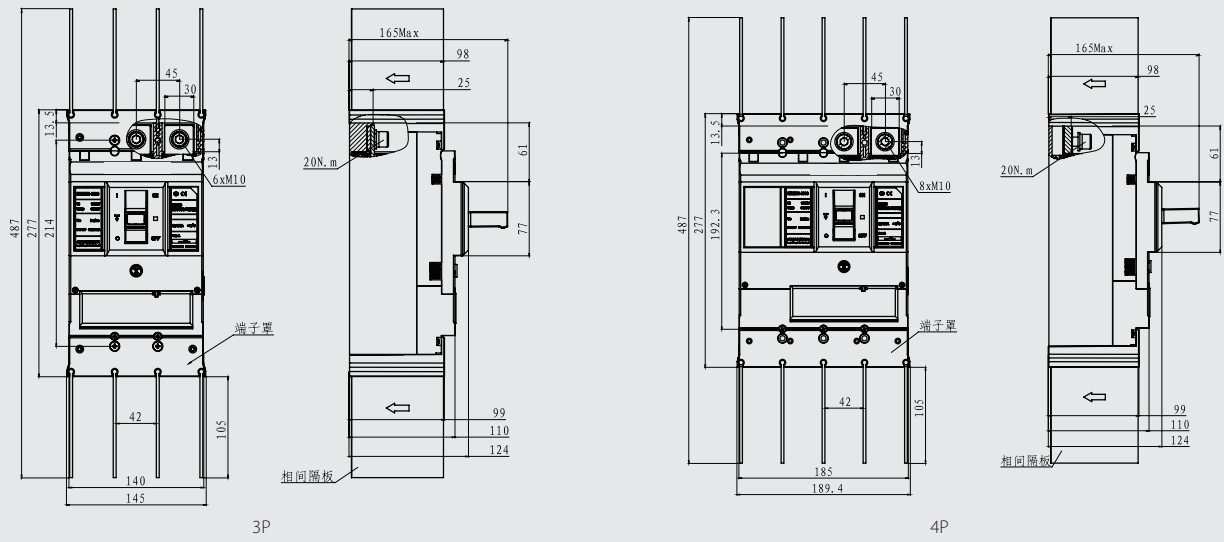
MDM5-400 二维图
