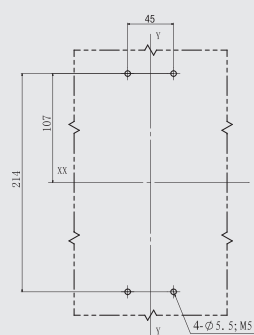
3P安装孔
