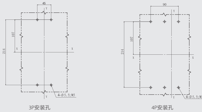
MDM5-400 二维图
