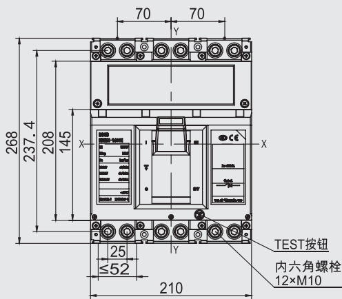
三板前接线外形尺寸
