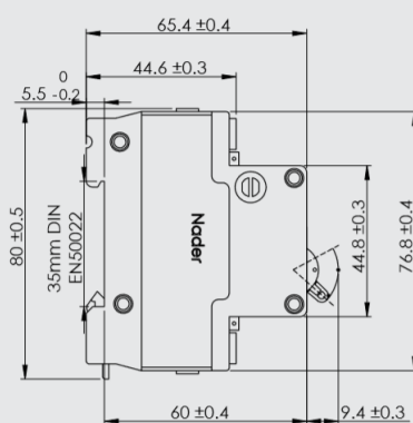
1P侧视图
