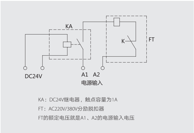
分励脱扣器瞬动电流及功耗
