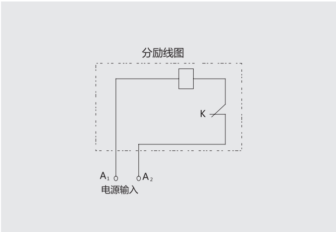
分励脱扣器接线图
