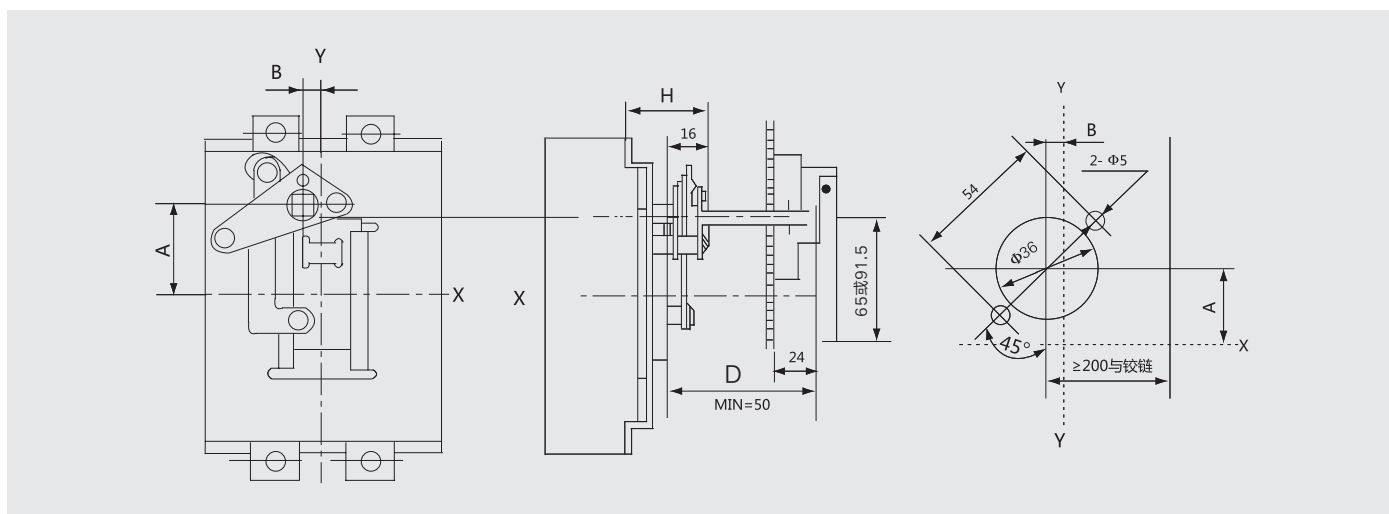
CS2-B型手柄安装开孔示意图
