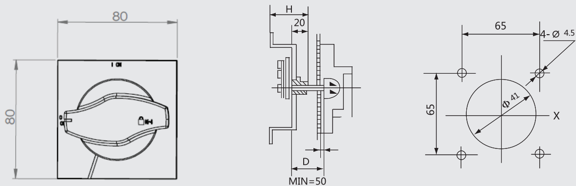
IP65手柄（250壳架以下）开孔示意图
