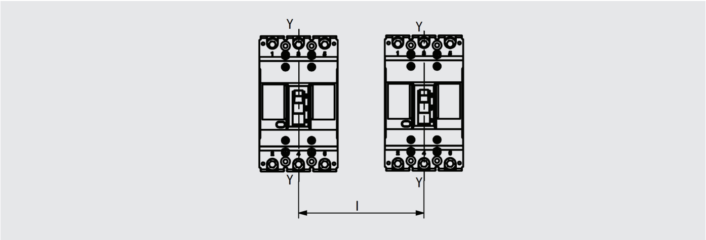
断路器排装间的最小中心距离
