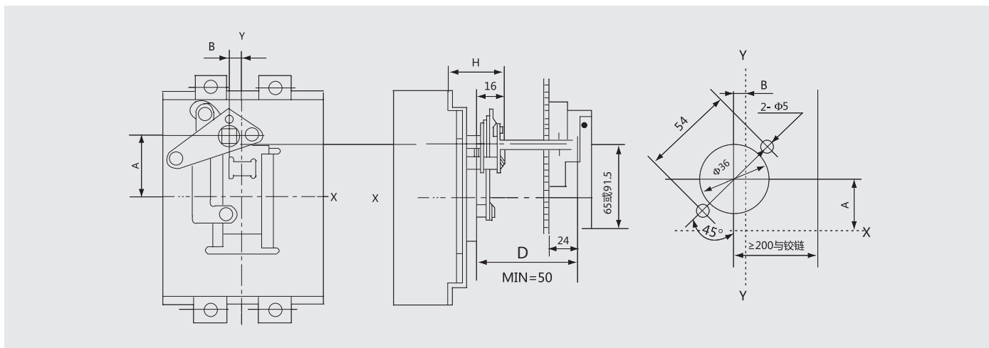
CS2-B型手柄安装开孔示意图
