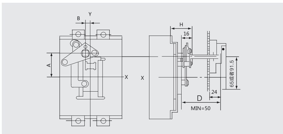
CS2-B型手柄安装开孔示意图
