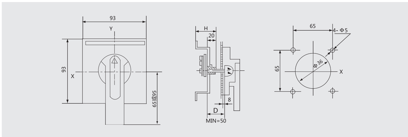
CS2-B型手柄安装开孔示意图
