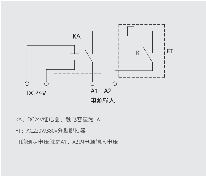
DC24V中间继电器配合AC220V/380V分励使用接线图
