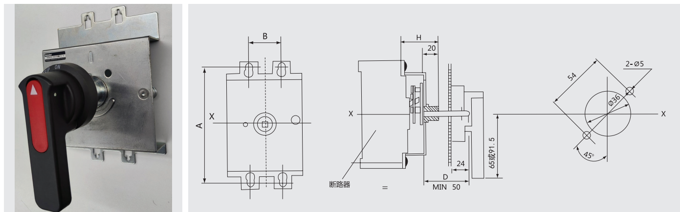
CS1-B型手柄安装开孔示意图
