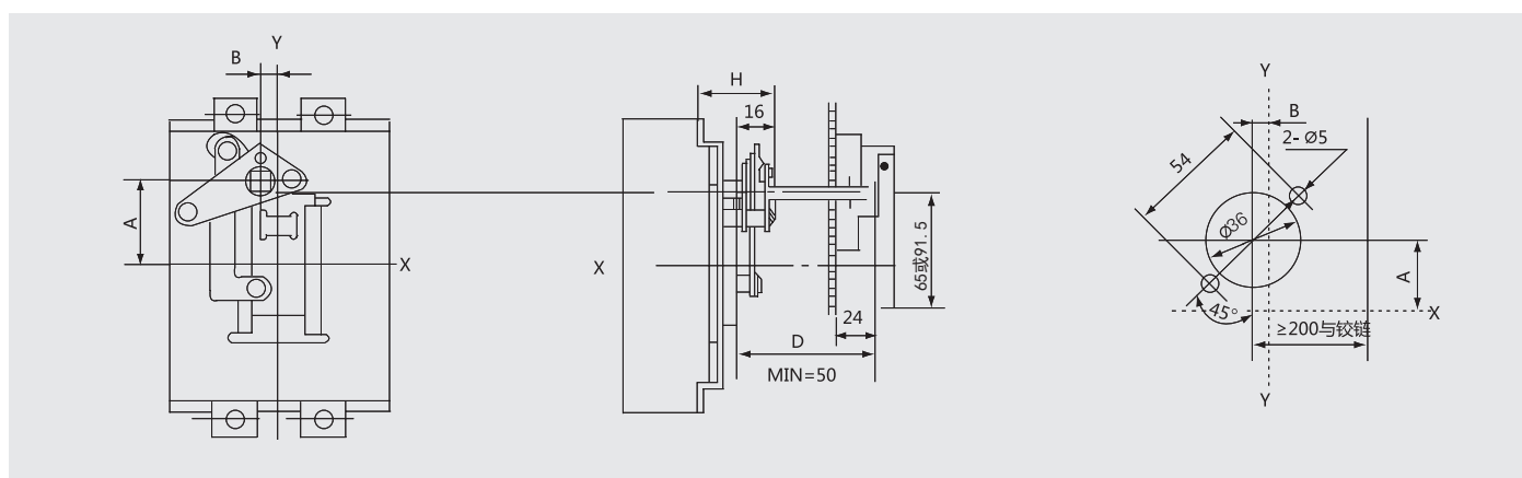
CS2-B型手柄安装开孔示意图
