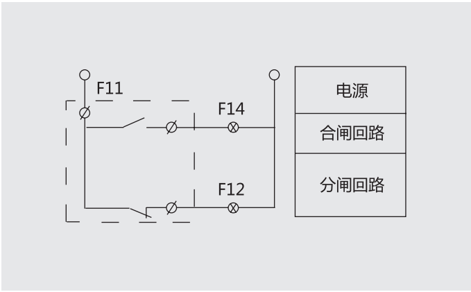
辅助触头接线图
