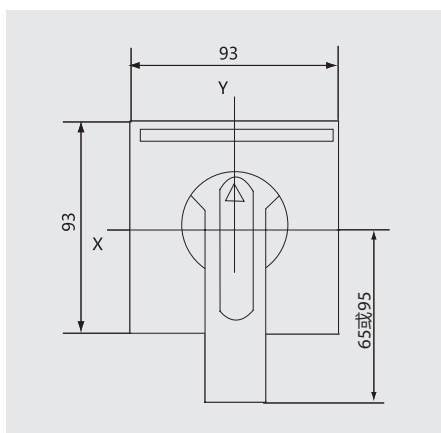
CS2-B型手柄安装开孔示意图
