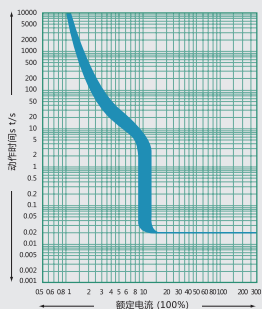
NDM3-400过载报警不脱扣特性曲线
