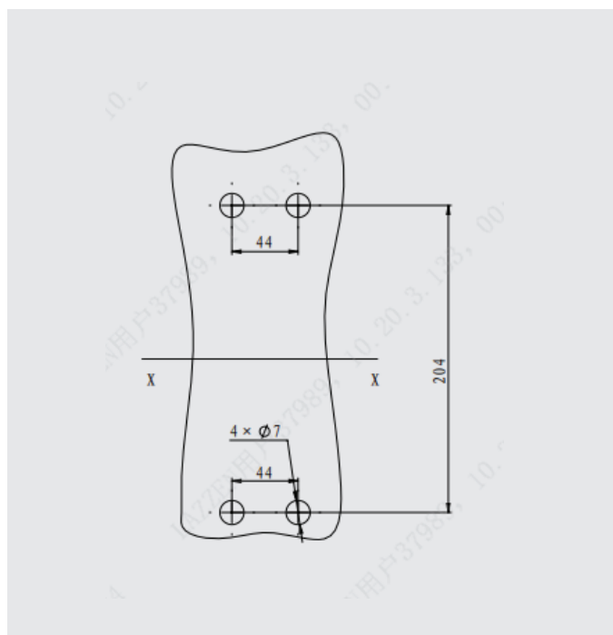
400/630-3P安装尺寸
