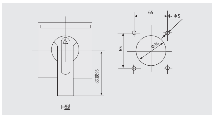
CS手动操作机构手柄安装开孔尺寸
