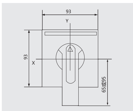
◆ CS2-B型手柄安装开孔示意图
