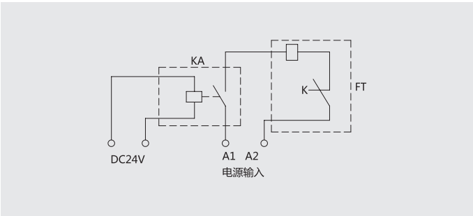
DC24V中间继电器配合AC220V/380V分励使用接线图
