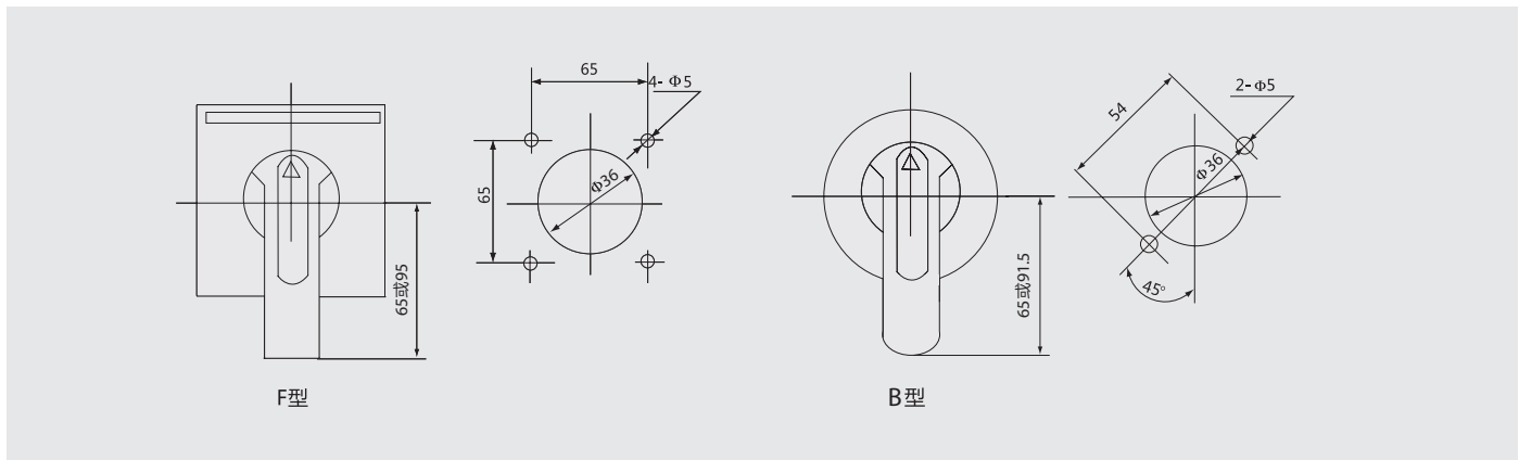
125/250/400/630手柄安装孔示意图
