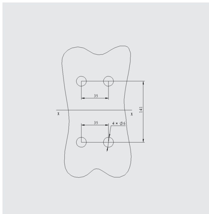
125/250-3P安装尺寸
