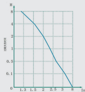
过载电流与失效时间特性曲线
