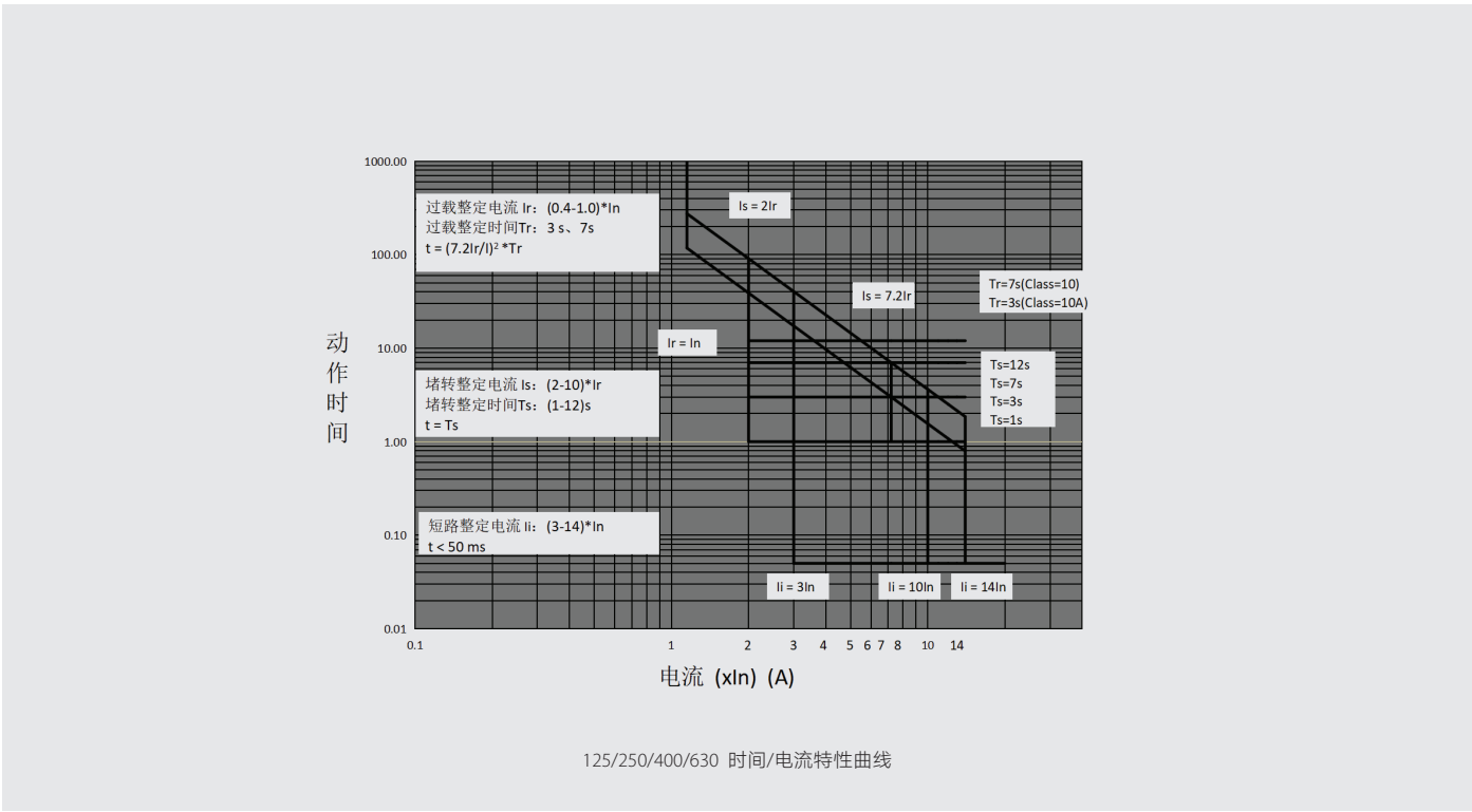
电动机型保护特性曲线
