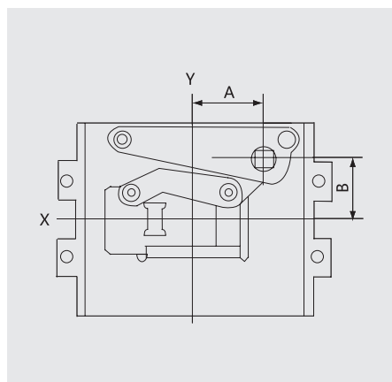
◆ IP65手柄（250壳架以下）开孔示意图
