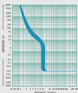
NDM3-250过载报警不脱扣特性曲线
