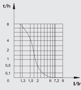
NDM3-400过载电流与失效时间特性曲线
