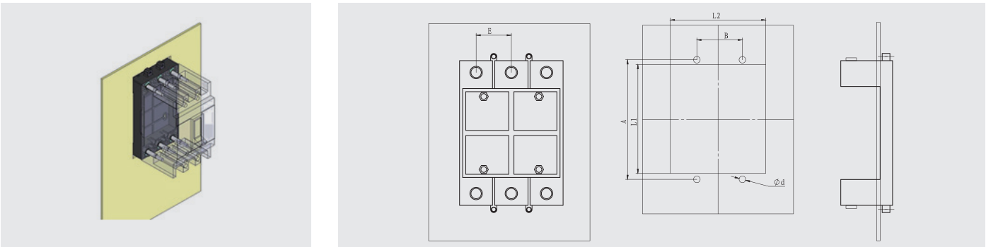
安装示意图
