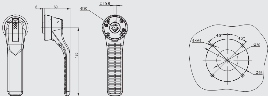
NDM3EX-1600 尺寸
