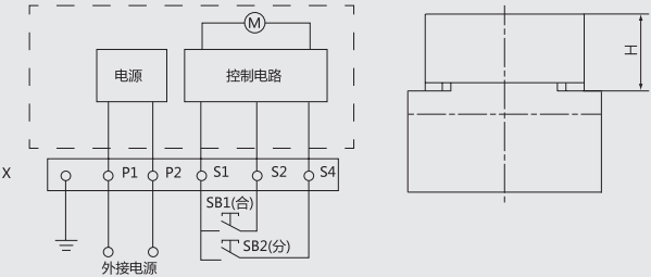
接线图（虚框内为断路器外部附件接线图）
