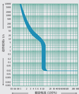
NDM3-630过载报警不脱扣特性曲线
