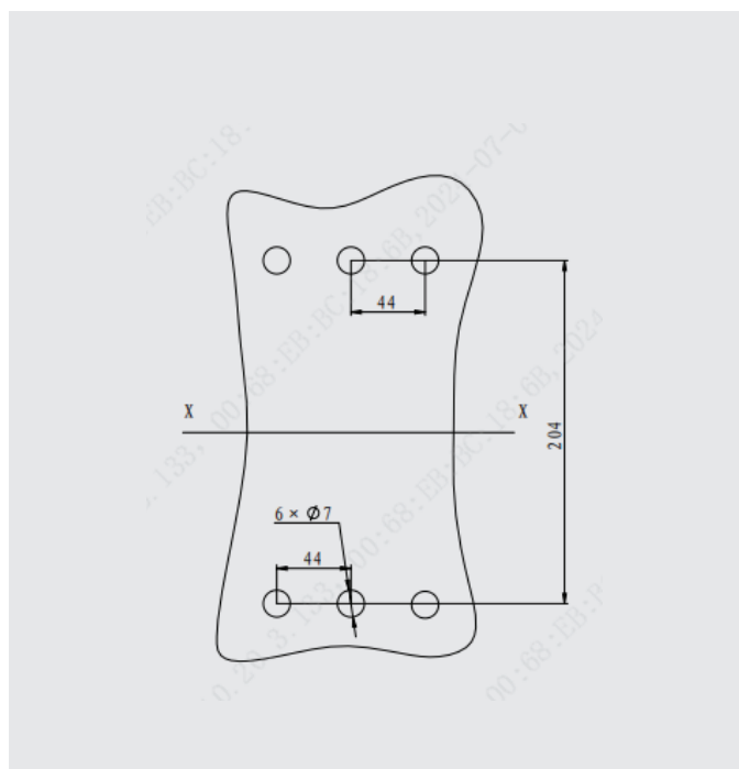
400/630-4P安装尺寸
