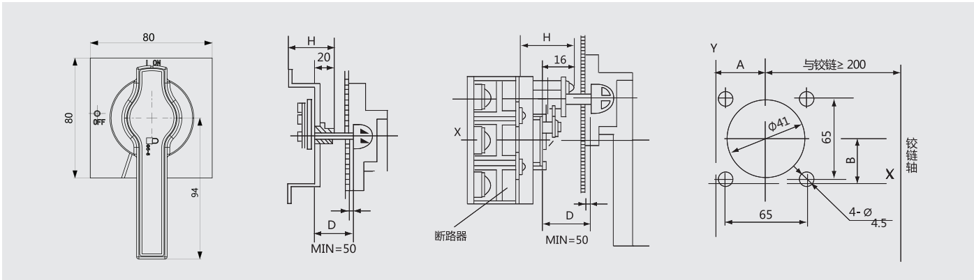
◆ 手动操作机构的安装方法及其外形尺寸
