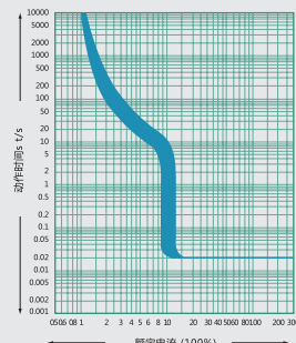
NDM3-630时间/电流特性曲线
