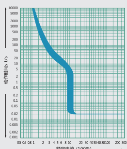
NDM3-125过载报警不脱扣特性曲线
