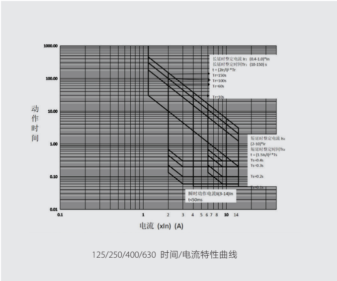
配电型长延时、短延时、瞬时保护特性曲线
