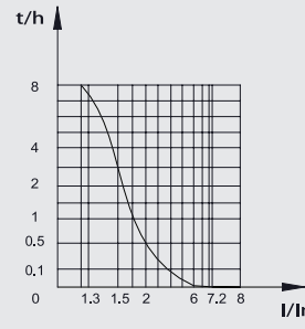
NDM3-630过载电流与失效时间特性曲线
