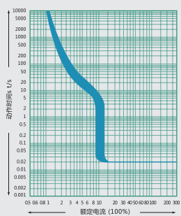
NDM3-400时间/电流特性曲线
