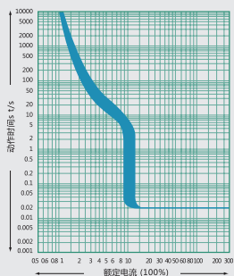
NDM3-250时间/电流特性曲线
