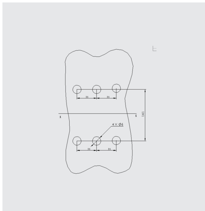
125/250-4P安装尺寸
