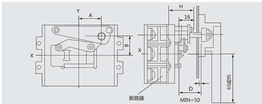
◆ CS2-F型手柄安装开孔示意图
