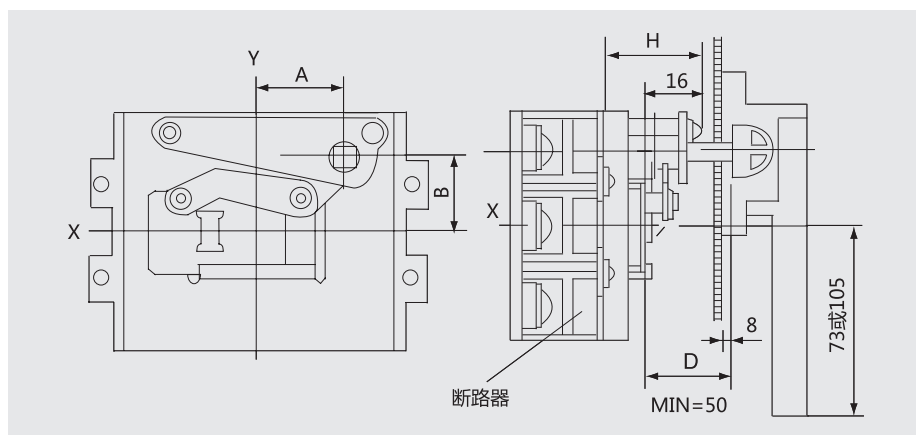
◆ IP65手柄（250壳架以下）开孔示意图
