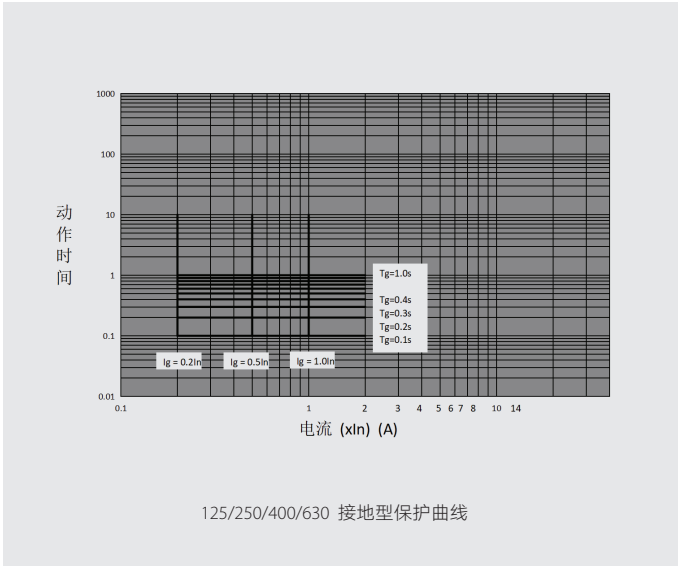
配电型接地保护特性曲线
