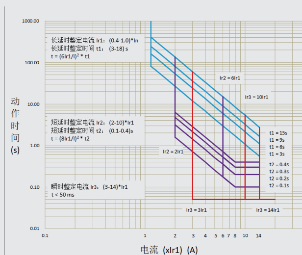
时间/电流特性曲线
