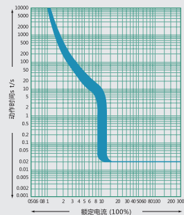
NDM3-800时间/电流特性曲线
