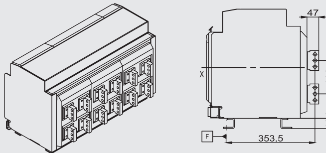
垂直接线
