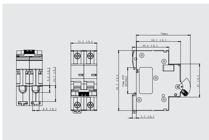
NDB2ZB-63外形尺寸
