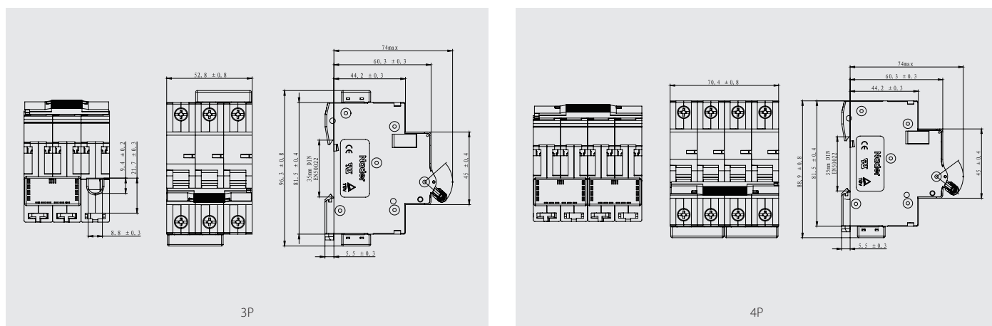
NDB2Z-63 (PV) 外形尺寸
