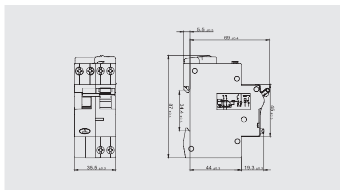
NDB2LE-40 外形尺寸
