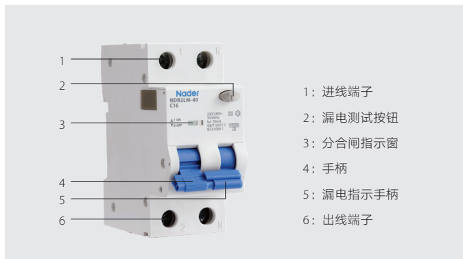
◆ NDB2LM-40外部结构图
