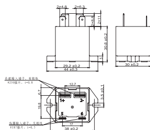
NDZ3X-40C
