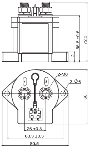
NDZ3W-250
