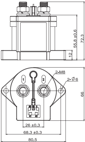
NDZ3W-150
