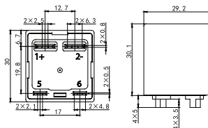
NDZ3X-20D
