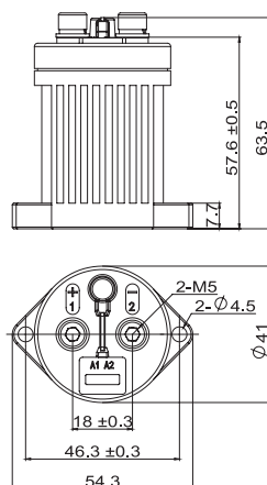
NDZ3-50
