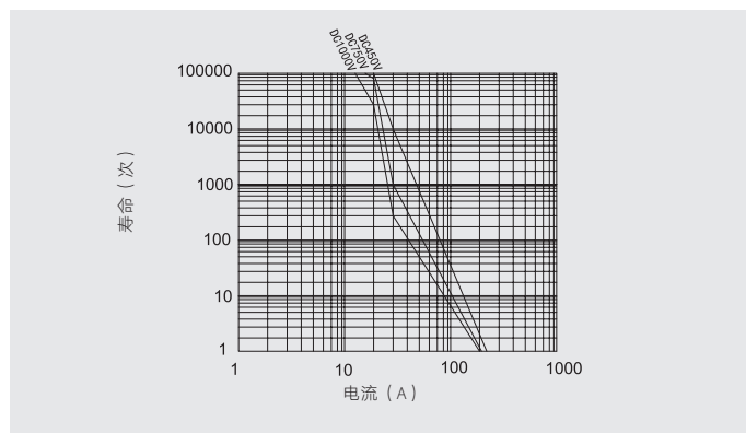
寿命曲线
