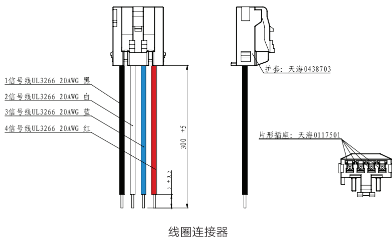
线圈连接器
