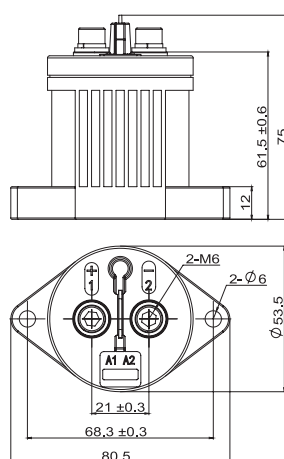
NDZ3-150
