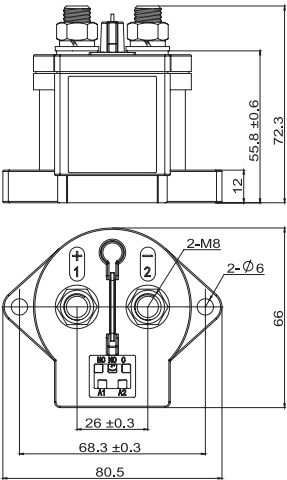
NDZ3X-250
