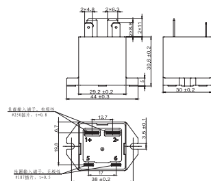
NDZ3X-20C
