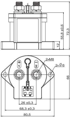
NDZ3-150J
