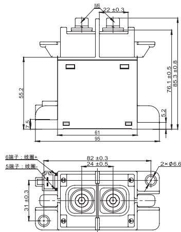
NDZ3T-200
