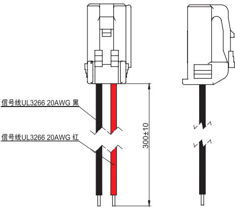
线圈连接器
