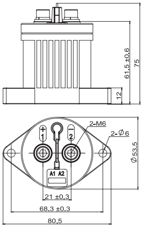
NDZ3X-150
