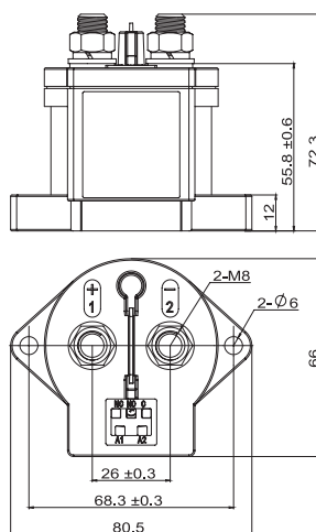
NDZ3-300
