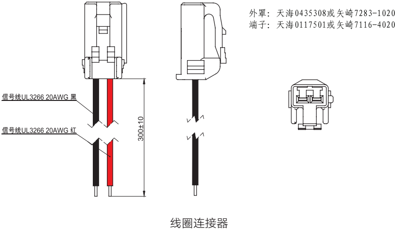
线圈连接器
