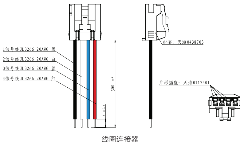
线圈连接器
