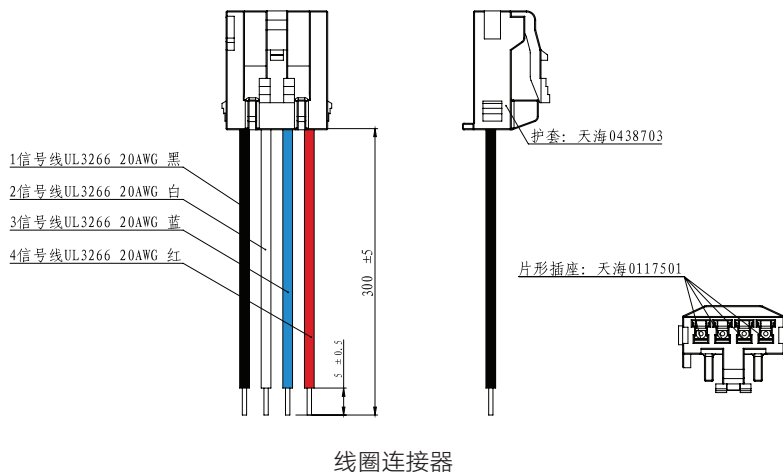
线圈连接器
