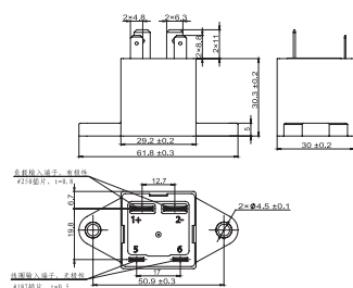
NDZ3X-40B
