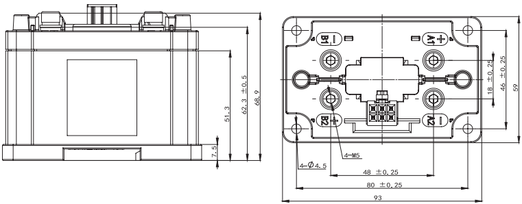
NDZ3X-100B/Z
