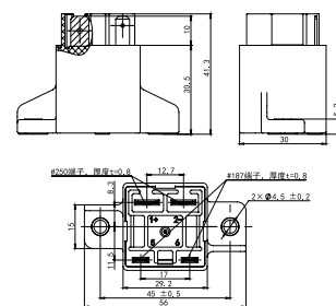
NDZ3X-40E
