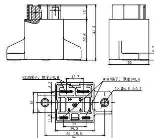
NDZ3X-20E
