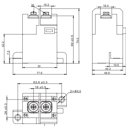
NDZ3T-150
