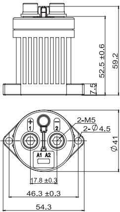
NDZ3X-100
