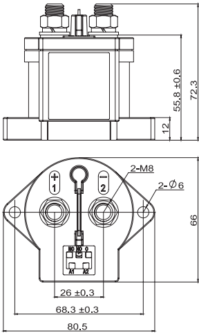
NDZ3-250
