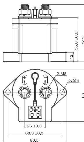
NDZ3X-150J
