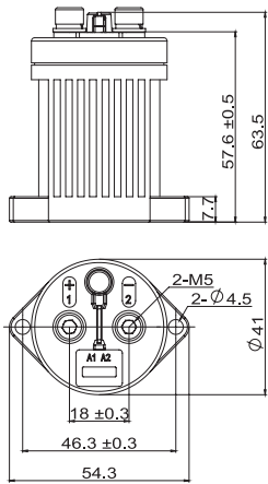
NDZ3-100
