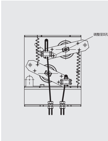
调整示意图
