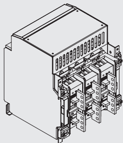
垂直接线
