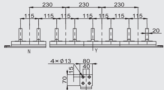
详图
