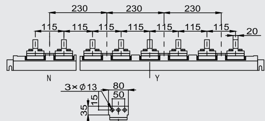
详图
