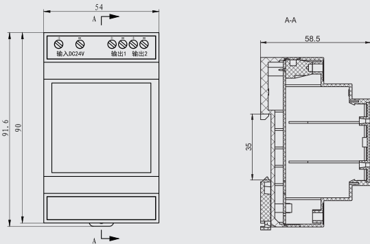
电源模块NWDF1-P1外形及安装尺寸图
