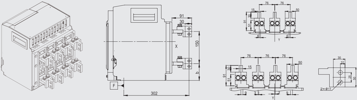
垂直接线
