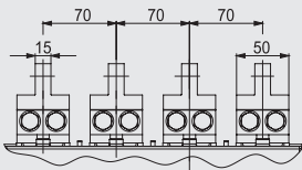
固定详图
