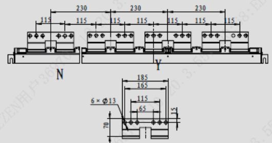
详图
