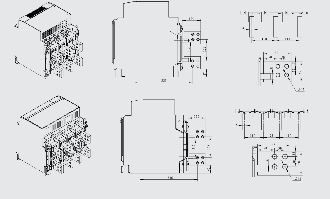
垂直加长接线
