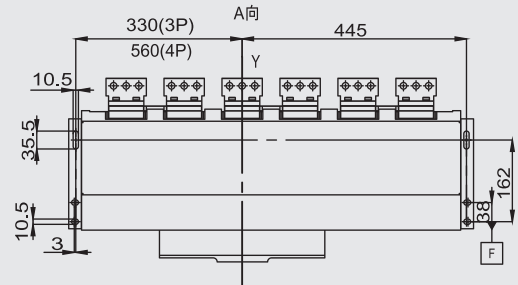
固定详图
