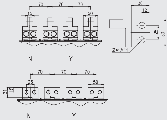
固定详图
