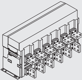
混合加长接线 (上水平下垂直)
