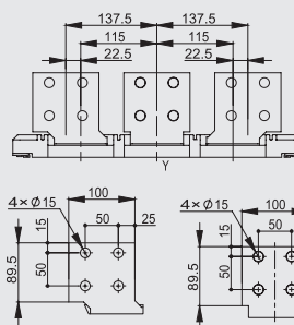
详图
