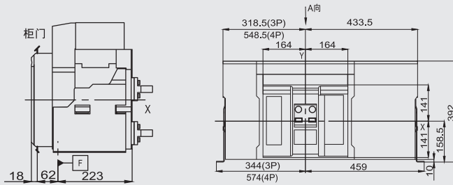
尺寸
