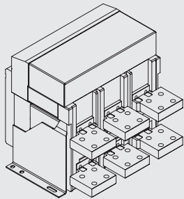
3200A-4000A水平加长、垂直加长接线
