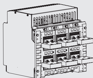
3200A-4000A水平加长、垂直加长接线
