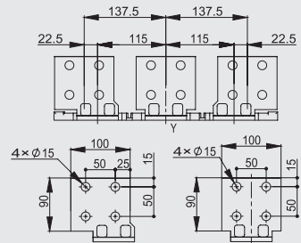
详图
