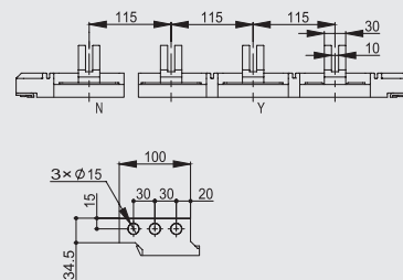
详图
