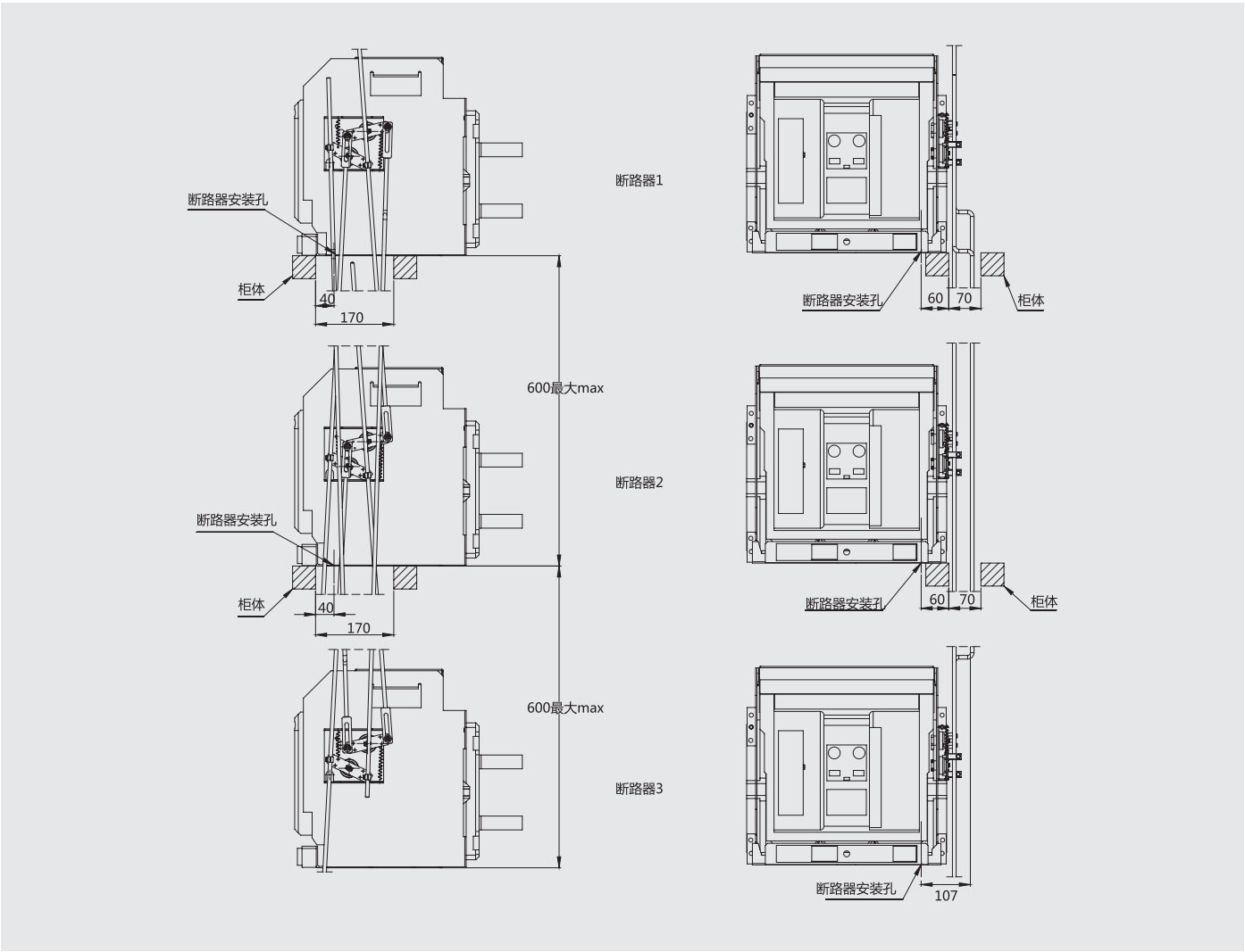
硬杆三联锁（一合两分） 安装示意图
