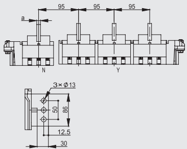
详图
