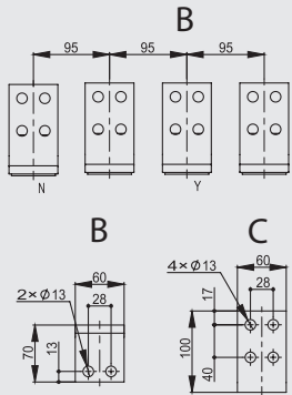
详图
