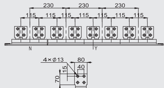
详图
