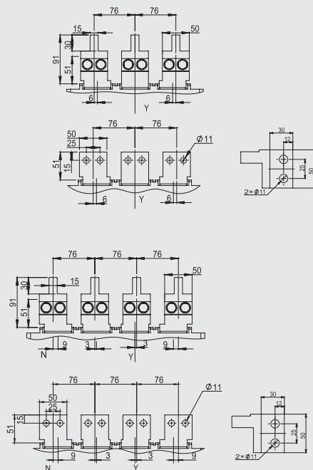
详图
