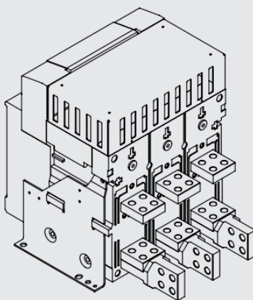
混合加长接线 (上水平、下垂直)
