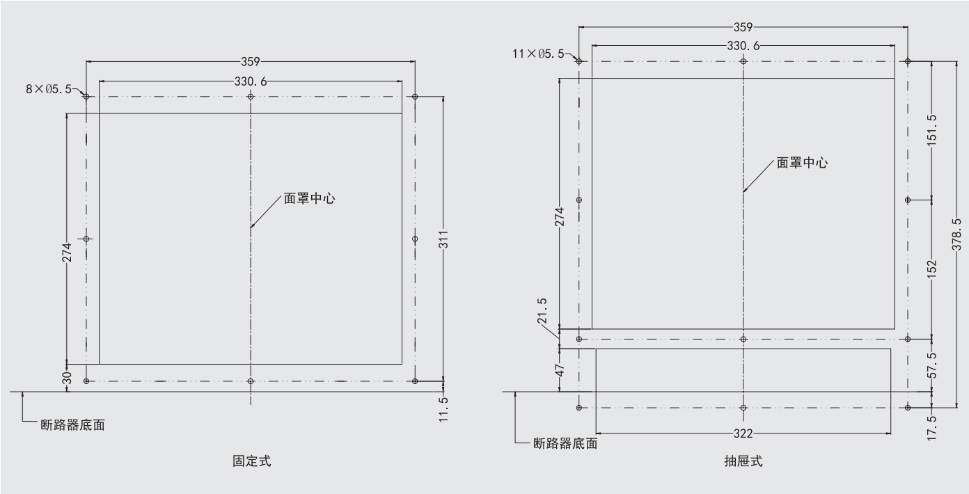
NDW1A-6300门框开孔尺寸 (单位: mm)
