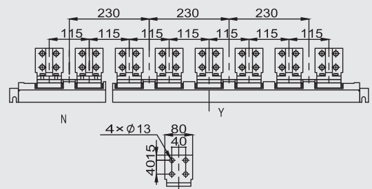
详图
