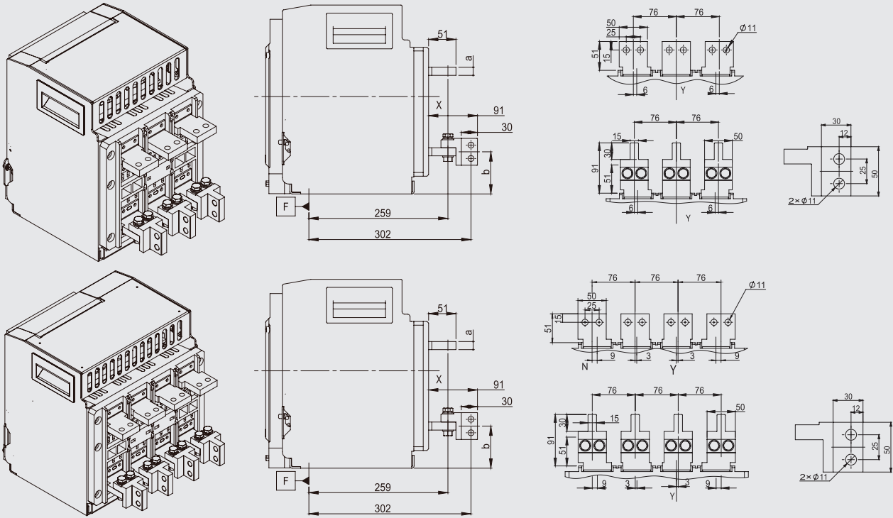
上水平下垂直接线
