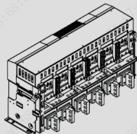
混合接线（上水平下垂直）
