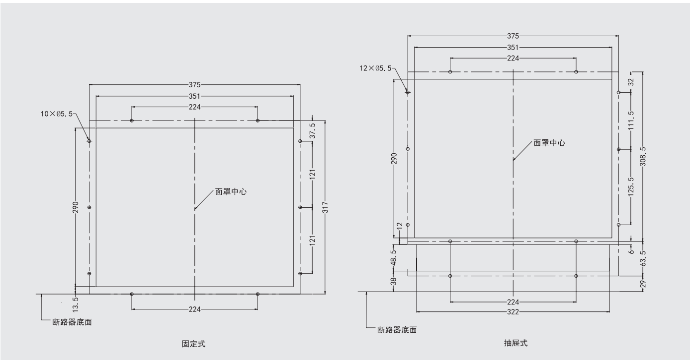
NDW1A-6300门框开孔尺寸 (单位: mm)
