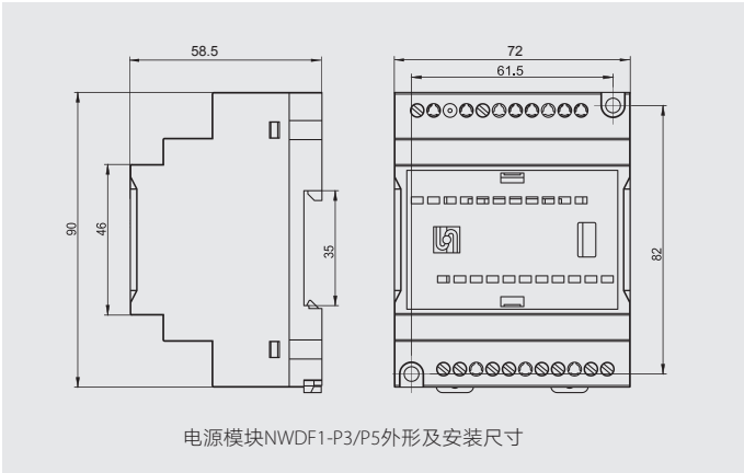
电源模块NWDF1-P1外形及安装尺寸图
