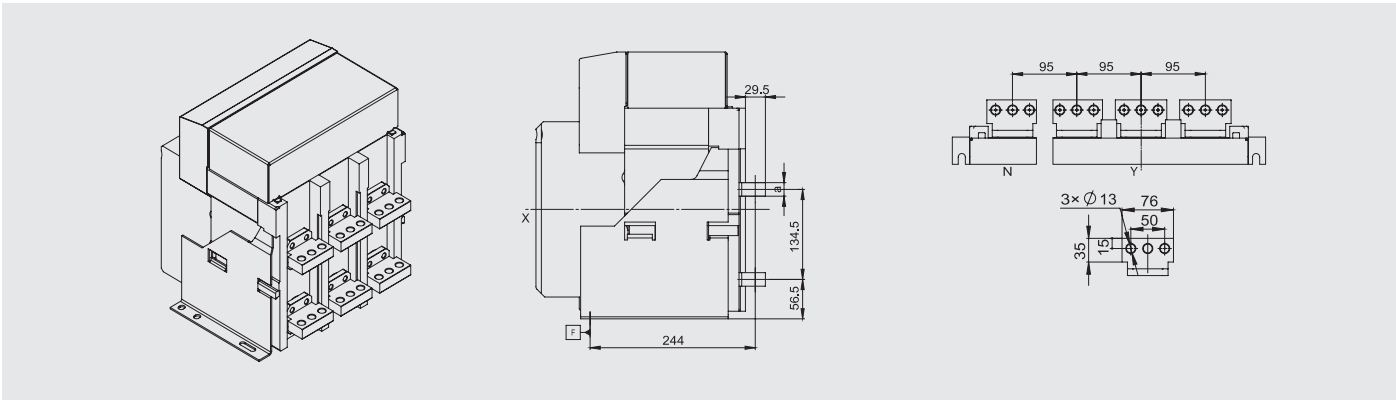
水平接线
